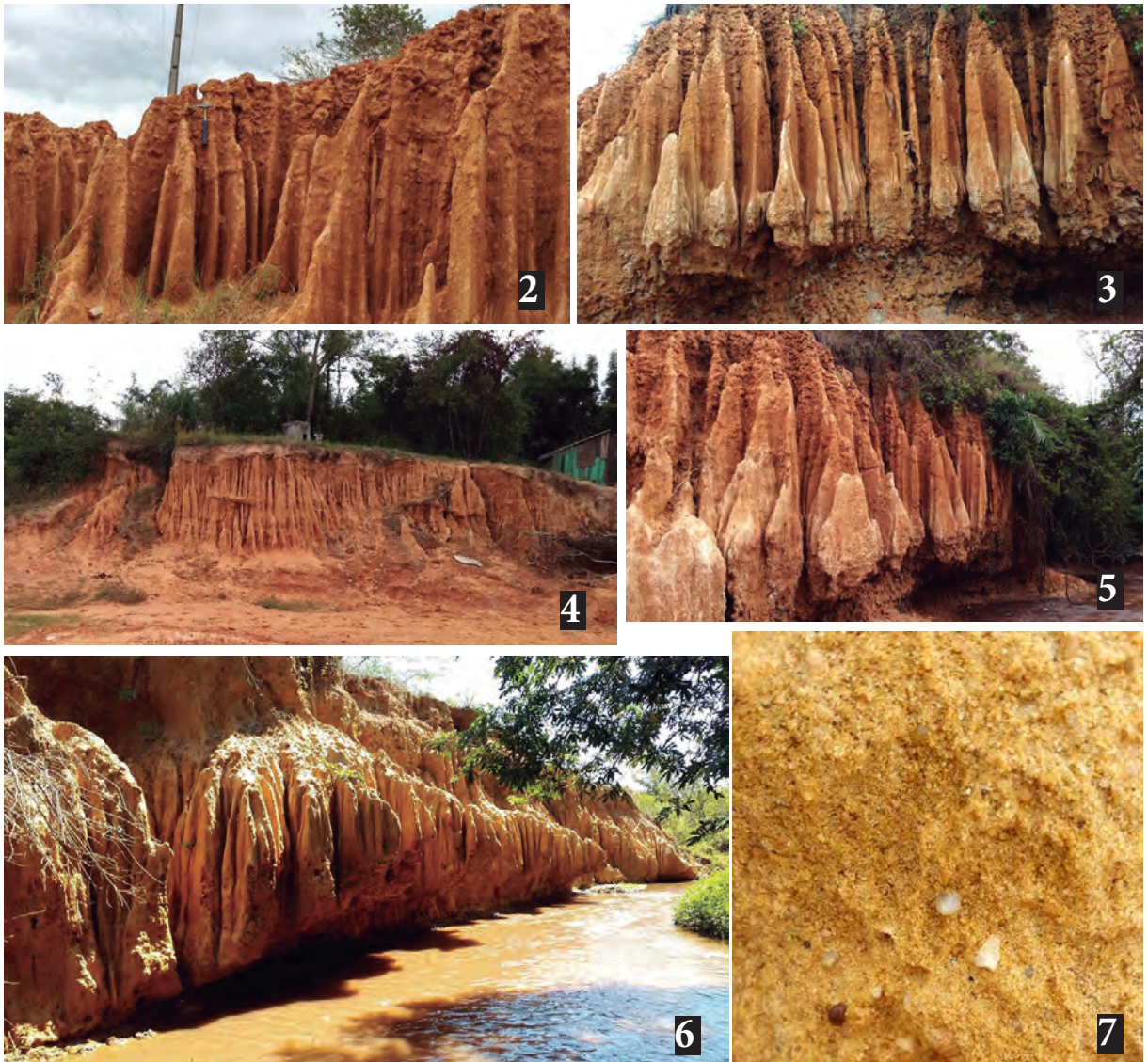
Figuras 2-7. Formaciones de “ badlands ” de la zona de Ypané. 2) “ Badlands ” en barranco alledaño al Arroyo Ypané en una de sus mejores exposiciones [25.463105°S; 57.526342°W]. 3) Los pináculos de “ Badlands ” de mayor longitud hallados al costado del Arroyo Ypané [25.463105°S; 57.526342°W]. 4) “ Badlands ” a ambas márgenes de un camino vecinal, camino al Río Paraguay. Se observa un desarrollo moderado en relación a aquellas localizadas en los barrancos del Arroyo Ypané [25.464676°S; 57.543977°W]. 5) Intensa erosión basal de los “ badlands ” en temporadas de crecidas del Arroyo Ypané. 6) “ Badlands ” en pa redones laterales del Arroyo Ypané [25.465442°S; 57.525963°W]. 7) Detalle de los sedimentos estudiados.
